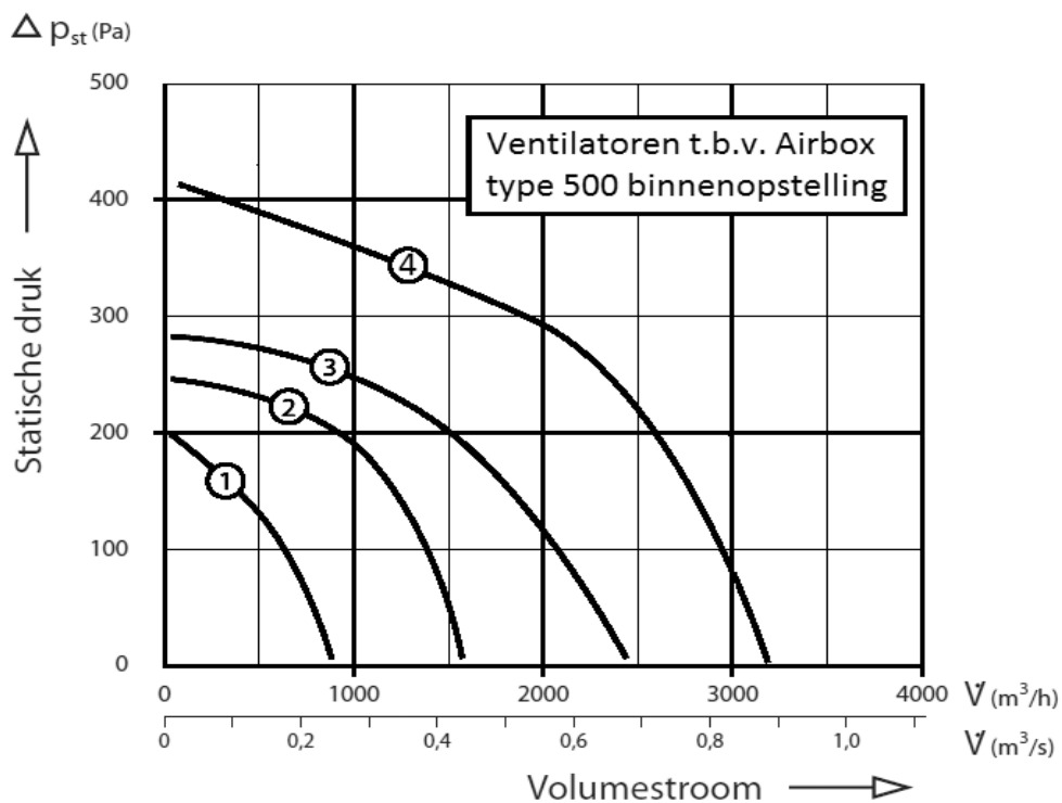
Airbox 500 binnenopstelling
